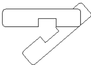
Principe du mi-bois
